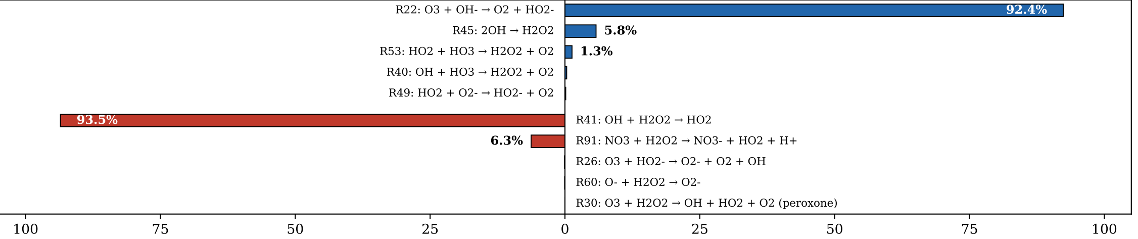
(d) H 2 O 2 (Σsrc = 2.16e-12 M/s)
